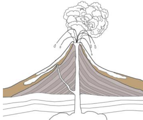
cône volcanique
