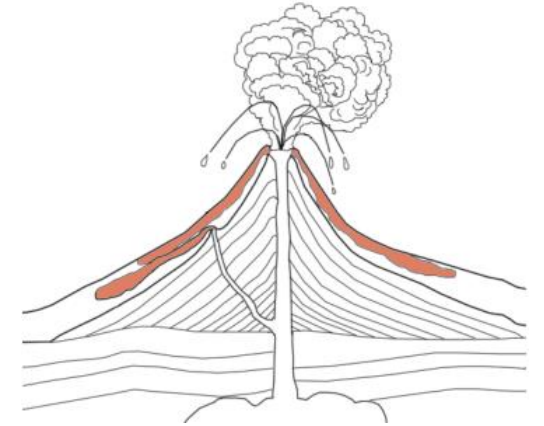
lave
