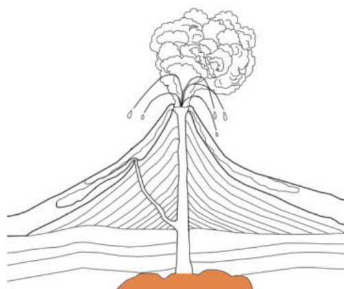
chambre magmatique
