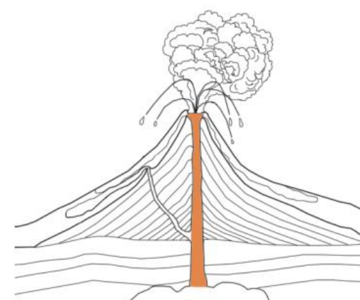
cheminée principale
