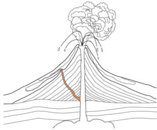
cheminée secondaire
