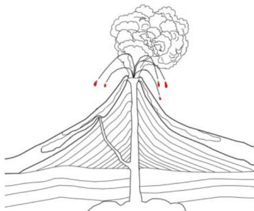
bombe volcanique
