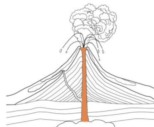
cheminée principale
