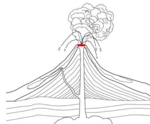
cratère
