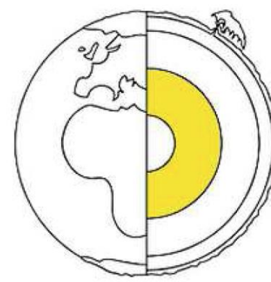
noyau externe
