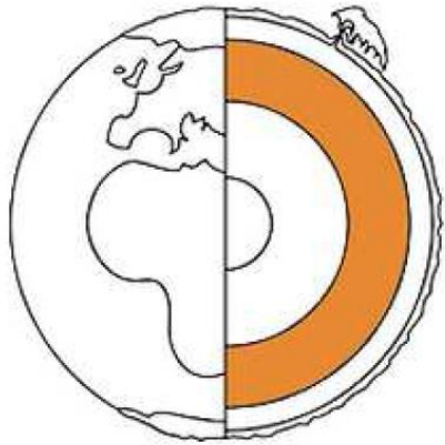
manteau inférieur
