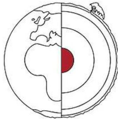
noyau interne
