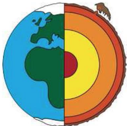
terre
