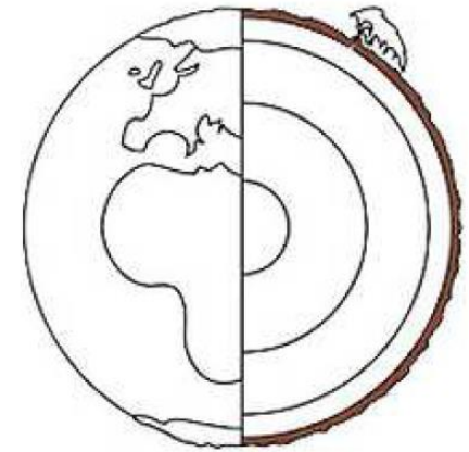
croûte terrestre
